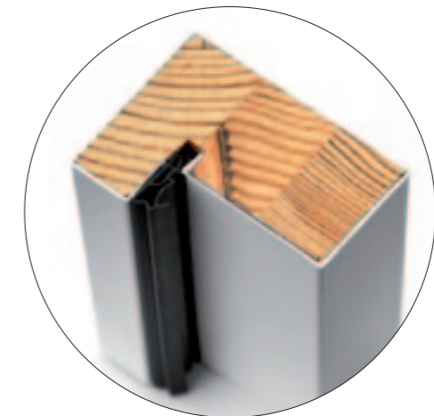
PRZEKRÓJ OŚCIEŻNICY
