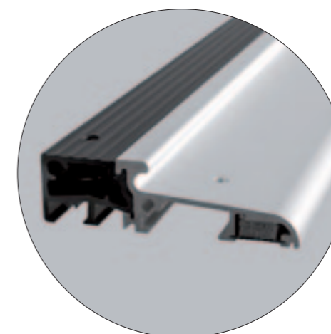
PRÓG ENERGO Z WKŁADKĄ TERMICZNĄ
