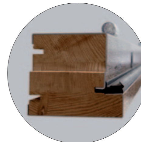
PRZEKRÓJ OŚCIEŻNICY
